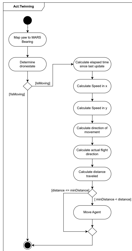
Abbildung 6.7: Aktivitätsdiagramm des Ablaufs des Twinning
